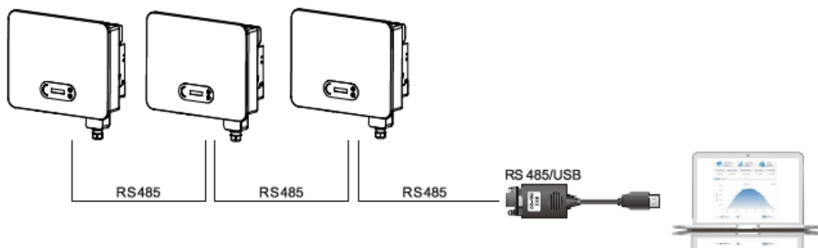
Rysunek 4-20: Podłączanie przewodów komunikacyjnych w przypadku wielu falowników SOFAR 15~24KTLX-G3 Zarejestrować funkcję zdalnego monitorowania urządzenia SOFAR 15~24KTLX-G3 w odpowiedniej witrynie internetowej lub aplikacji zgodnie z numerem seryjnym urządzenia do monitorowania.
