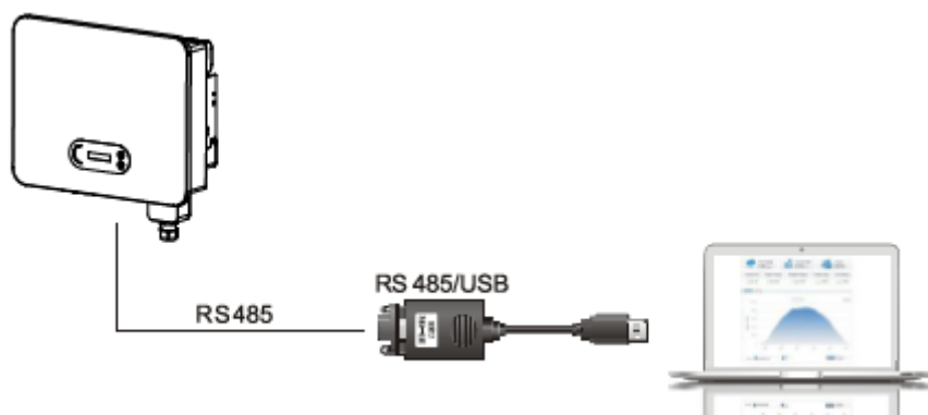
Rysunek 4-19: Podłączanie przewodów komunikacyjnych w przypadku pojedynczego falownika SOFAR 15~24KTLX-G3
