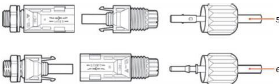
Rysunek 4-14 Podłączanie przewodu prądu stałego (4)
