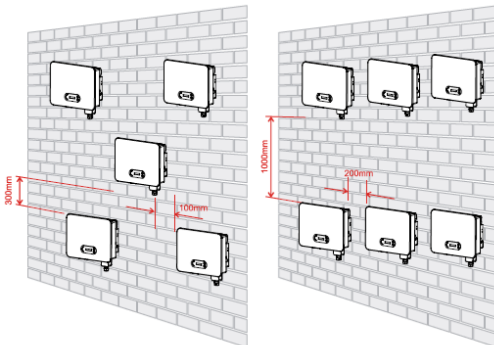
Rysunek 3-3: Odległości montażowe w przypadku wielu falowników
