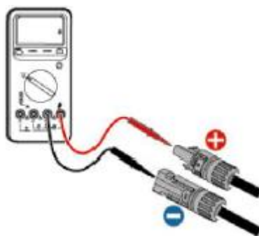
Rysunek 4-15: Dodatnią i ujemną elektrodę należy sprawdzić przy pomocy miernika uniwersalnego.
