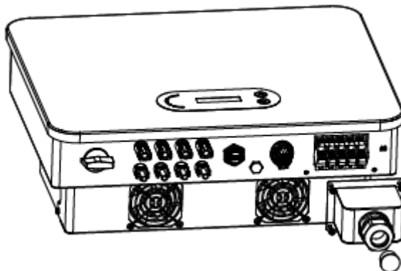
Rysunek 4-8: Schemat demontażu wodoszczelnej pokrywy złącza zasilania sieciowego
