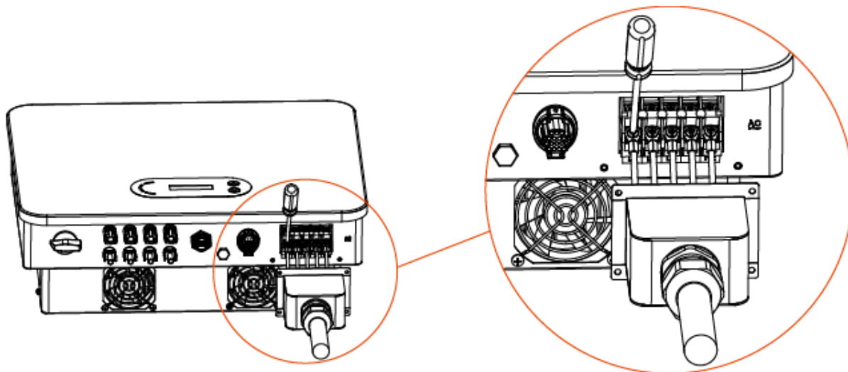
Rysunek 4-10: Schemat ilustrujący instrukcję podłączania przewodu zasilania sieciowego (2)
