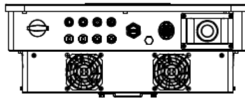
Rysunek 2-4b: Widok dolnej części urządzenia (20~24K)
