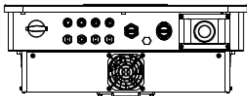
Rysunek 2-4a: Widok dolnej części urządzenia (15~17K)
