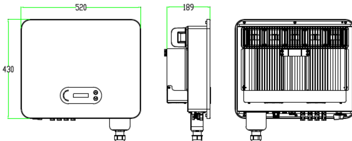
Rysunek 2-3: Widok urządzenia z przodu, z boku i z tyłu (15~24K)
