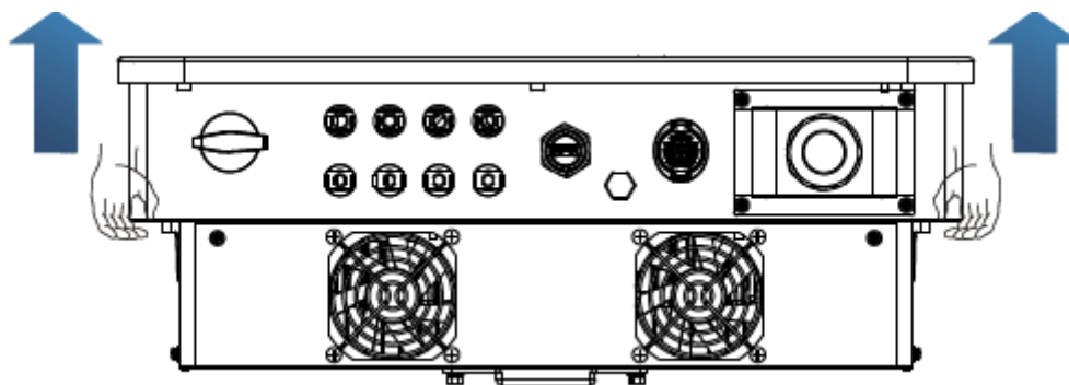
Rysunek 3-6: Wyjmowanie falownika z opakowania (2)
