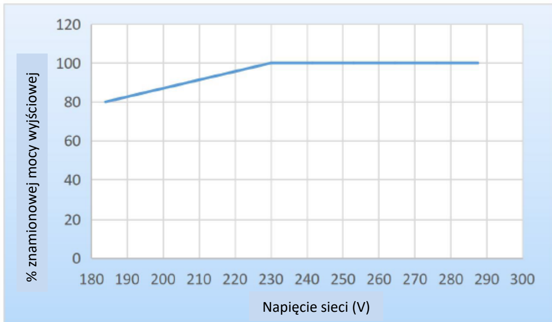
Rysunek 2-10: Zależność mocy znamionowej od napięcia sieci
