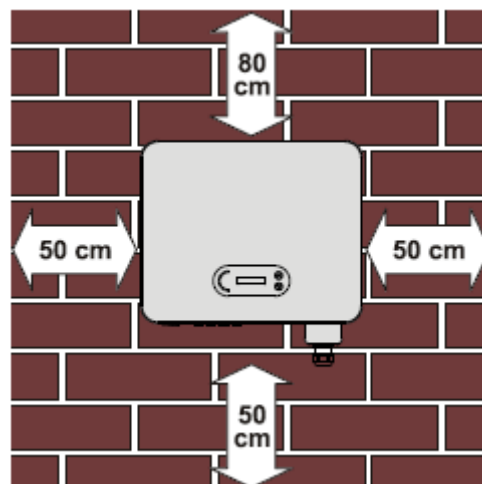
Rysunek 3-2: Odległości montażowe w przypadku pojedynczego falownika
