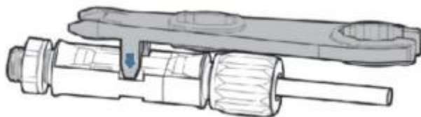
Rysunek 4-16: Odłączanie złącza prądu stałego
