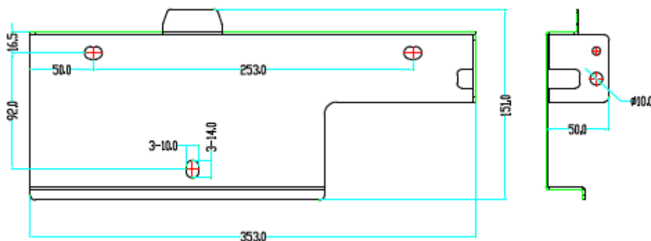
Rysunek 2-5: Wymiary wspornika
