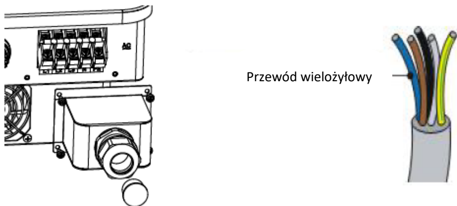
Rysunek 4-7: Złącze zasilania sieciowego SOFAR 15~24KTLX-G3
