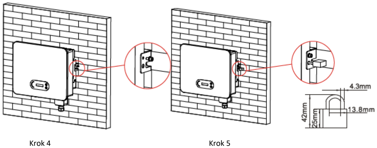
Rysunek 3-8: Instrukcja montażu (2)
