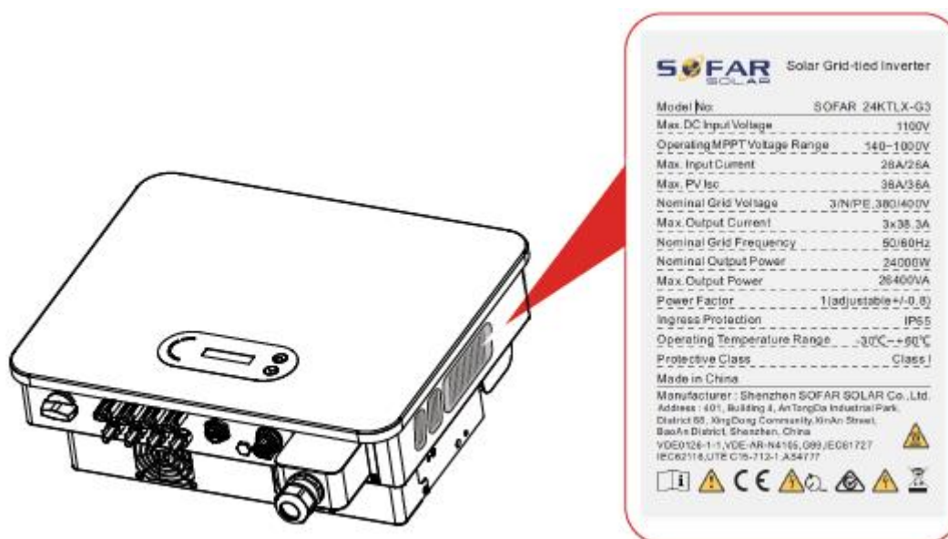
Rysunek 2-7: Etykieta produktu
