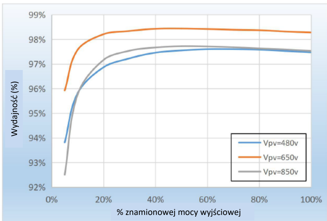
Rysunek 2-9: Krzywa wydajności (na przykładzie 20 kW)
