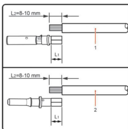
Rysunek 4-11: Podłączanie przewodu prądu stałego (1)
