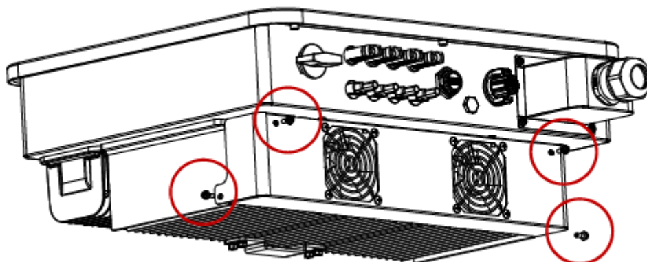
Rysunek 7-1: Usunąć cztery śruby z panelu wentylatora.
