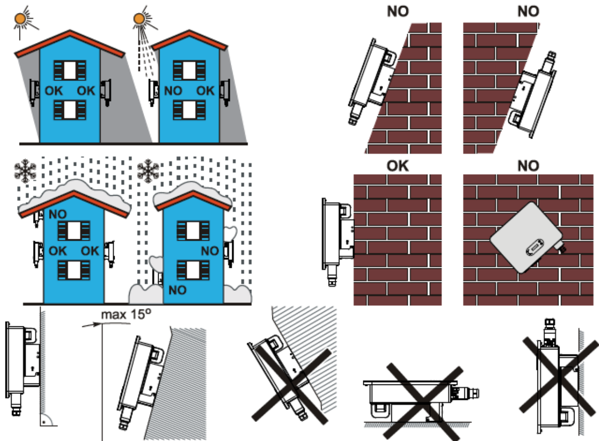
Rysunek 3-1: Wybór położenia montażowego
