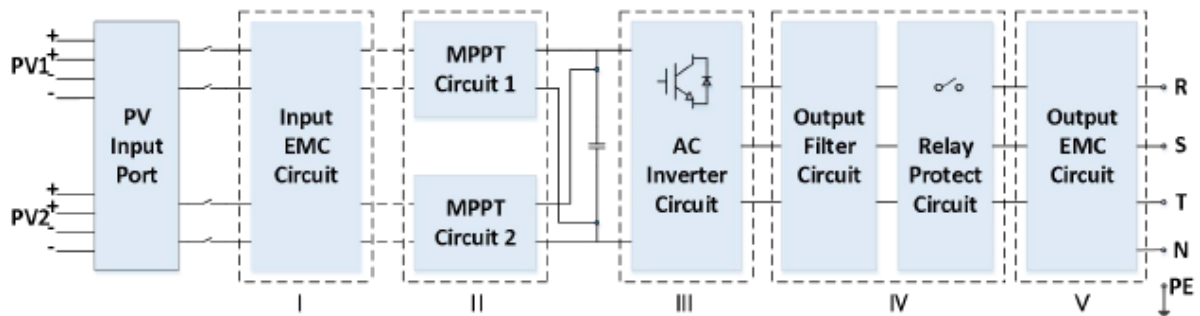
Rysunek 2-8: Schemat połączeń elektrycznych
