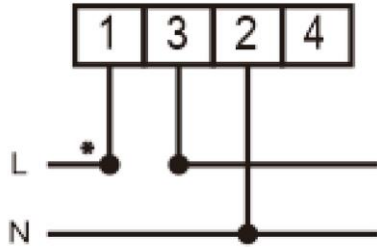
Modo de conexión: 1 Fase 2 Hilos
